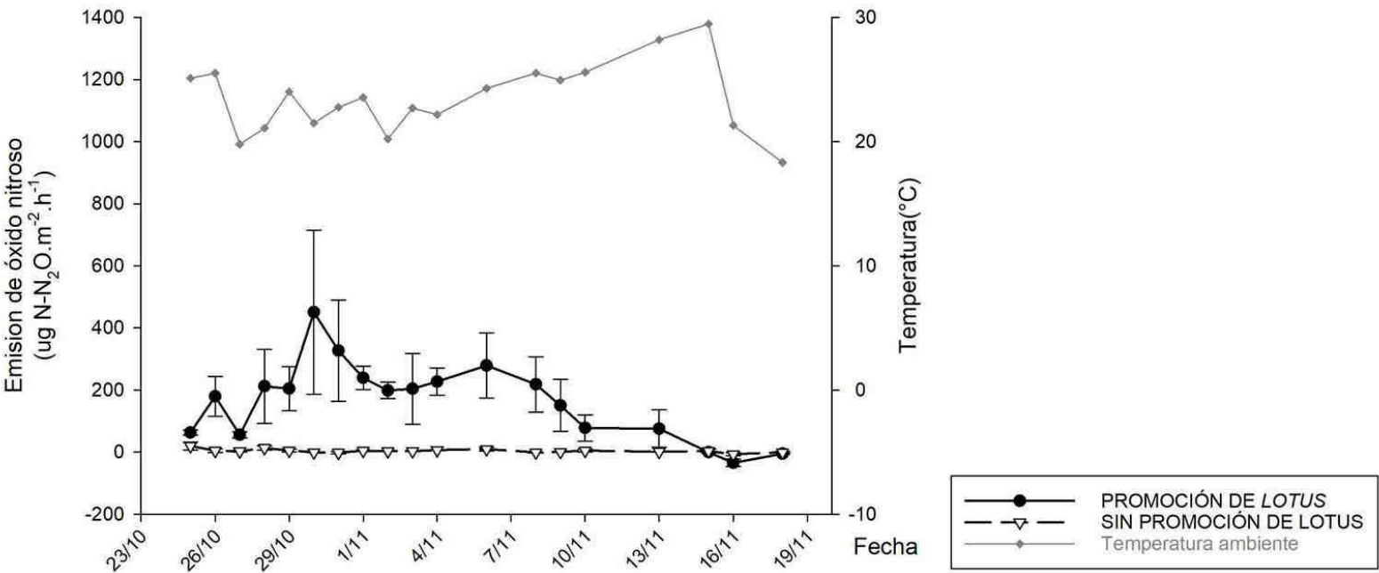
Emisiones primaveral de óxido nítrico (N 2 O) en sistemas pastoriles con y sin promoción de Lotus tenuis .
